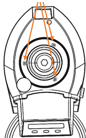
MOLLE REGOLAZIONE MACINATURA
